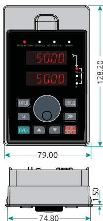
Рисунок 2-13. Установочные размеры LED-пульта управления
