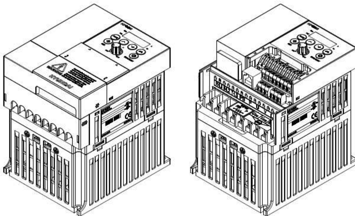
Рис. 1-4 Внешний вид инвертора N700E (2 конструкция)
