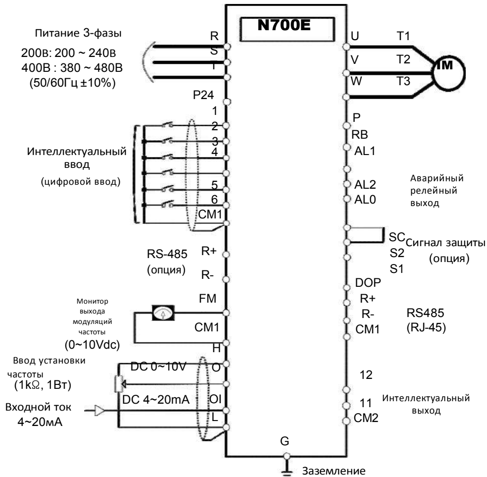
Рис. 3-1 Схема настройки при помощи управления клеммами.
