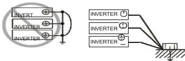
Рис. 2-3 3 Заземление (G)
