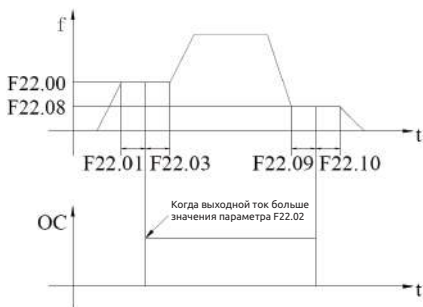
Рис. 7-51. Процесс отпущания тормоза при подъеме
