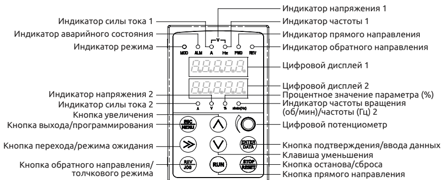
Рис. С-1. Устройство панели управления EN-LED4
