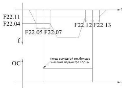
Рис. 7-52. Процесс отпущания тормоза при опускании
