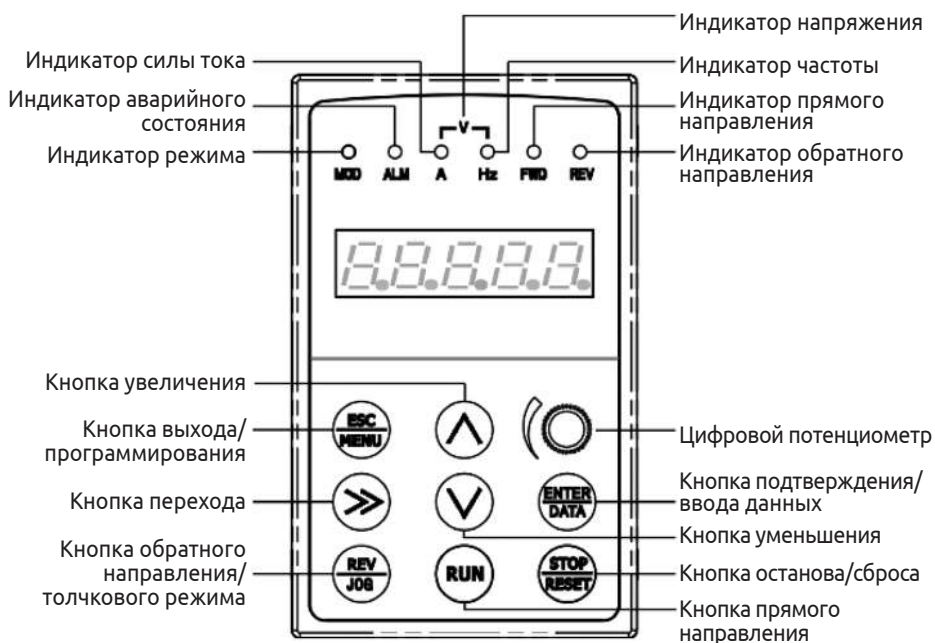
Рис. 5-2 Устройство панели управления
