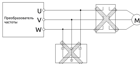
Рис. 3-6 Запрет на использование контактора и фильтрующего конденсатора
