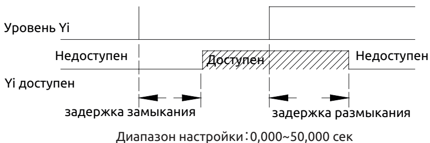
Рис. 7-30 Принцип действия многофункциональной выходной клеммы
