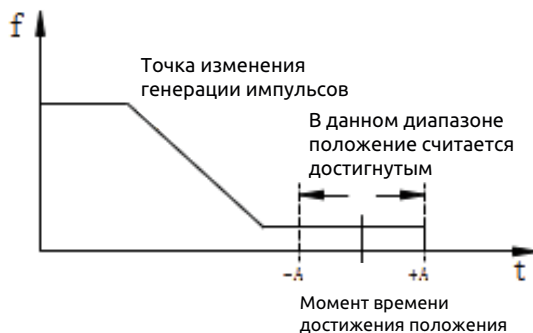
Рисунок 7-45. Достижение диапазона настройки при позиционировании
