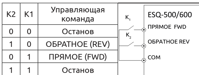
Рис. 7-16 Режим двухпроводного управления 1
