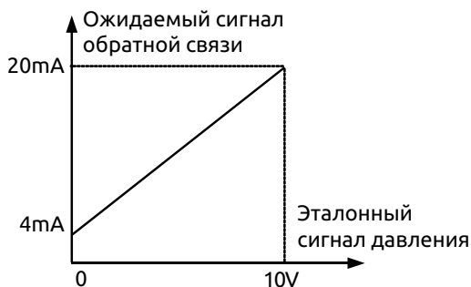
Рис. 7-38 Эталонный и ожидаемый сигнал обратной связи
