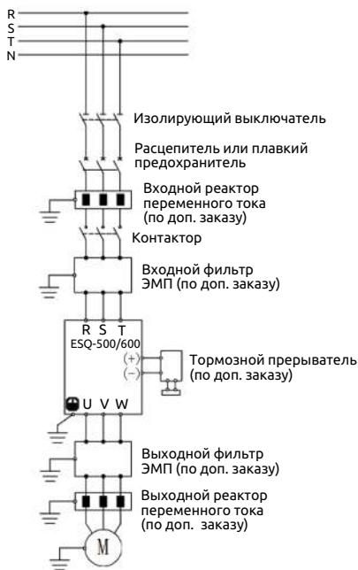
Рис. 3-8 Подключение различных устройств к преобразователю
