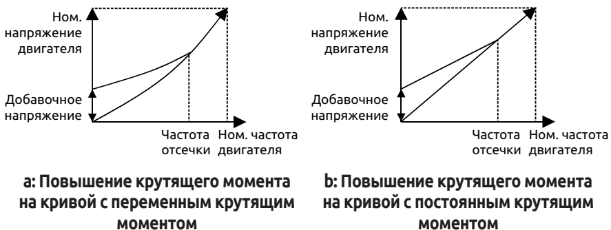
Рис. 7-8 Повышение крутящего момента
