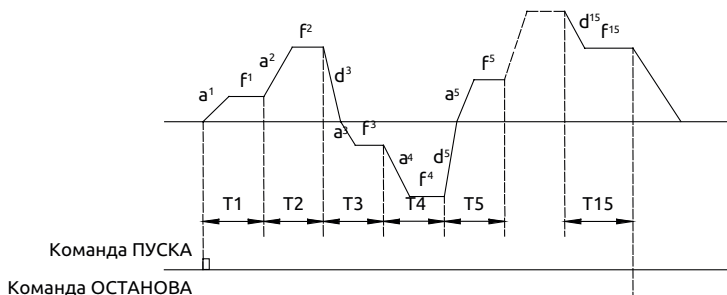
Рис. 7-31 Останов ПЛК после завершения одного цикла
