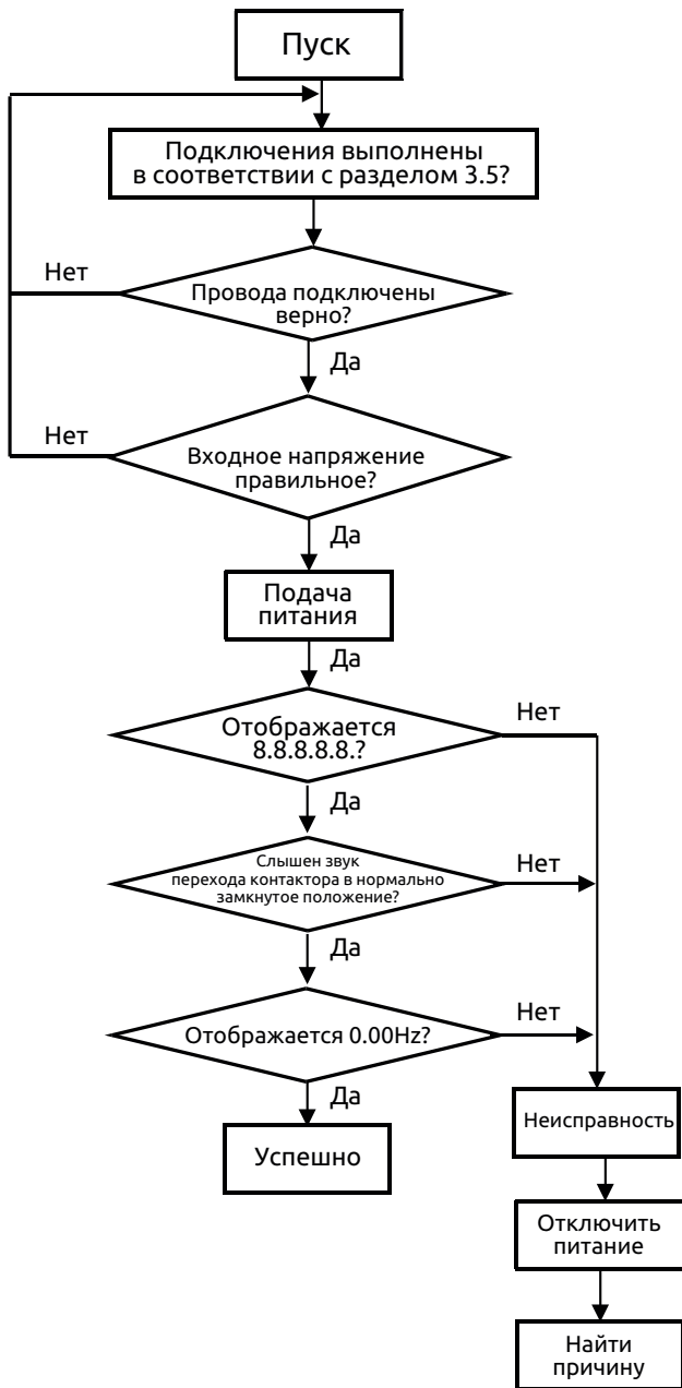
Рис. 5-12 Порядок действий при первом включении питания
