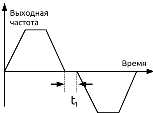
Рис. 7-6 Время простоя при переключении на ПРЯМОЕ/ОБРАТНОЕ вращение
