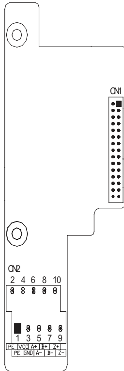
Рис. E-1. Чертеж плат EN-PG01, EN-PG02
